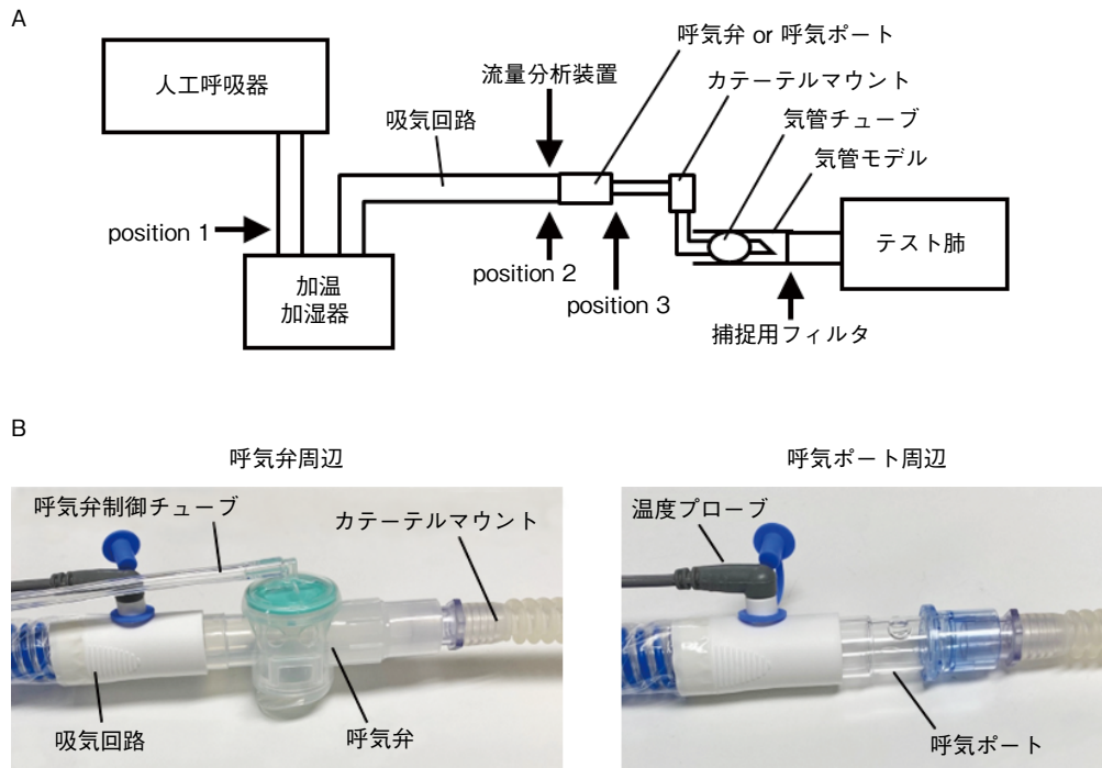
図1 人工呼吸器シングル回路（呼気弁回路または呼気ポート回路）における振動メッシュ式ネブライザ（vibrating mesh nebulizer : VMN）のサルブタモール送達率および換気パラメータ測定の実験回路
