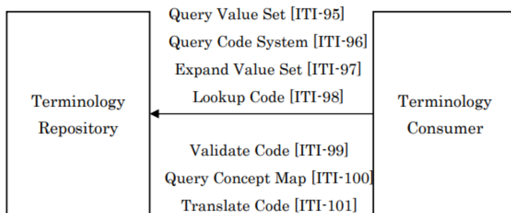
図2 値セット、コード、マップの共有(SVCМ)のアクタとトランザクション
