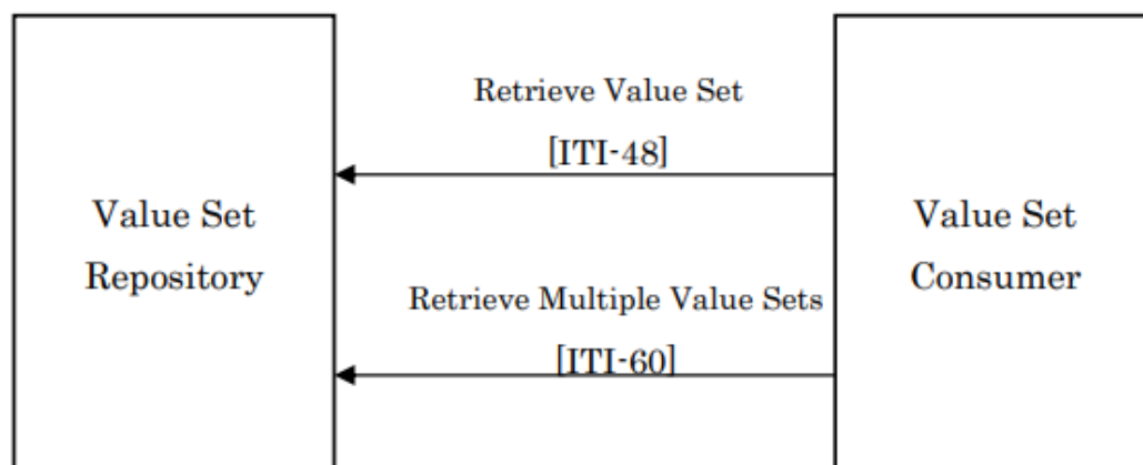
図1 値セット共有(SVS)のアクタおよびトランザクション
